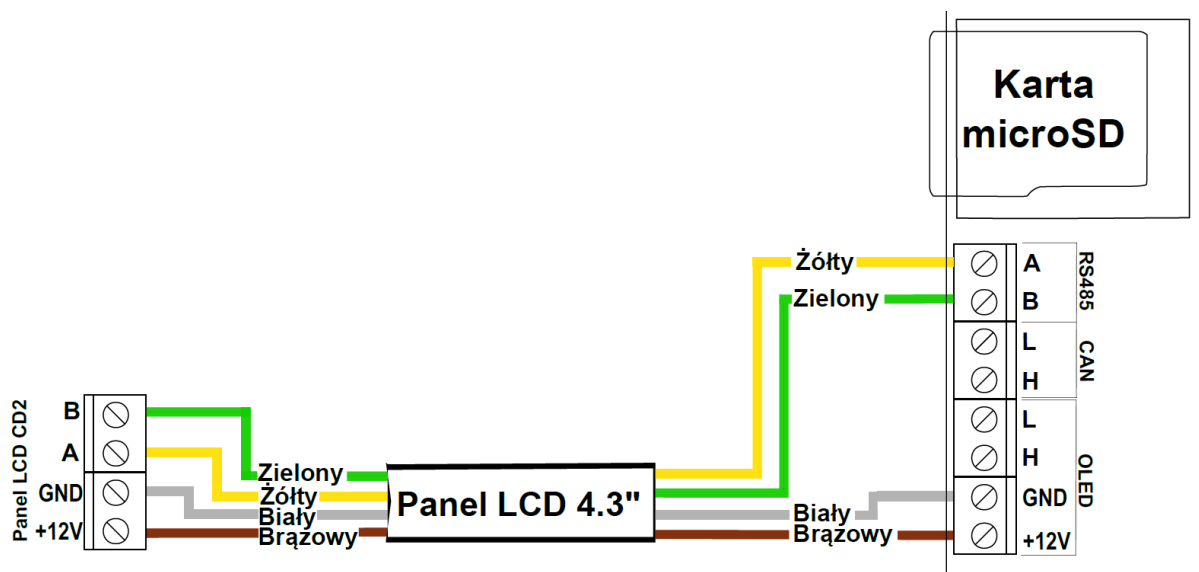
Ilustracja 2: Podłączenie panelu CD2/CD3 4.3" w sterowniku v3.5
