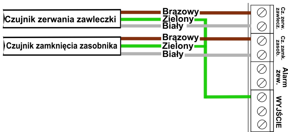
Ilustracja 3: Podłączenie czujników: zerwania zawleczki oraz zamknięcia zasobnika
